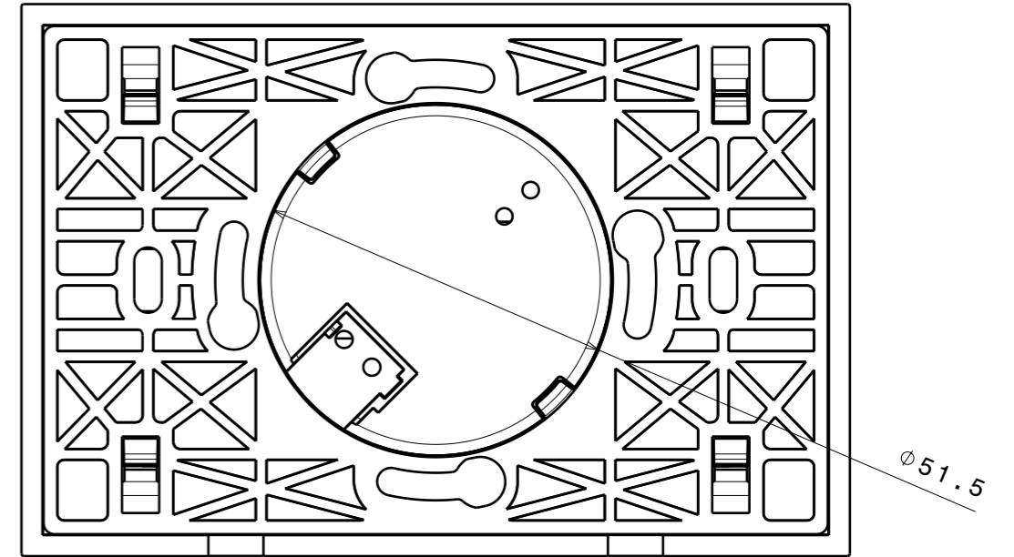
Vista dal basso Scala: 1:1
