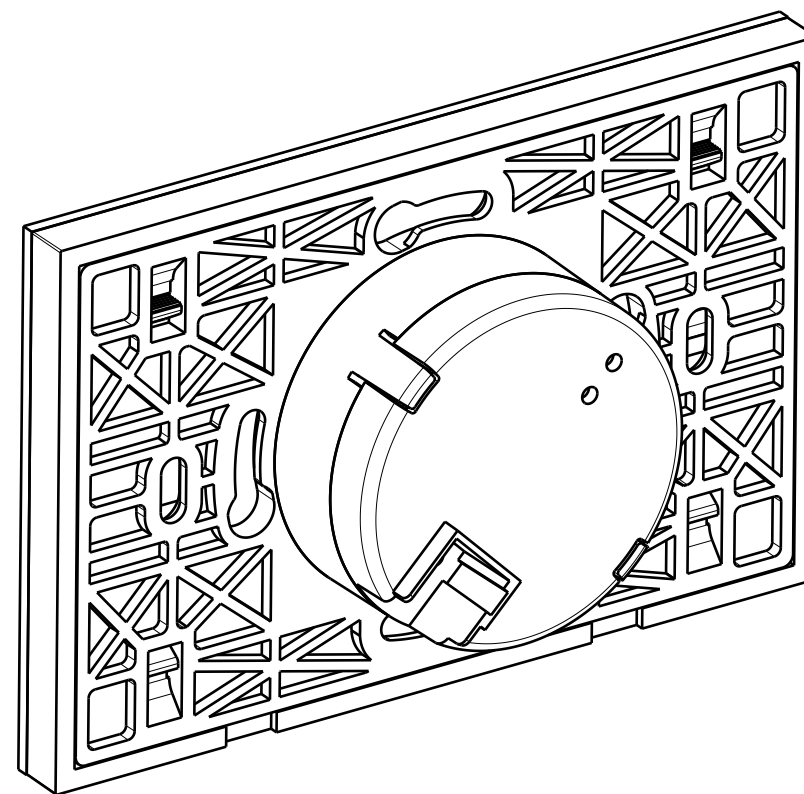
Vista isometrica Scala: 1:1
