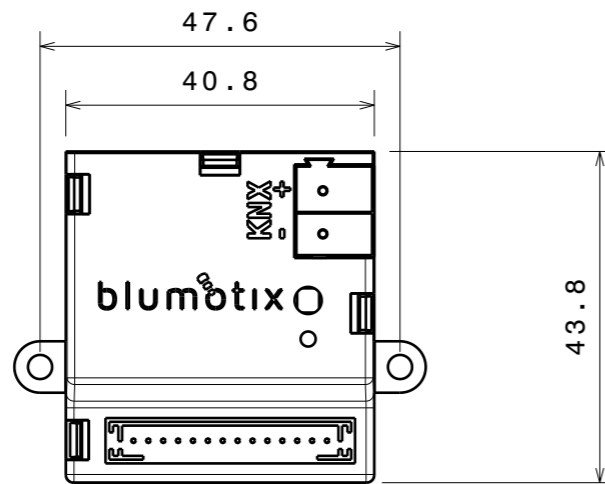
Vista dall'alto Scala: 1:1
