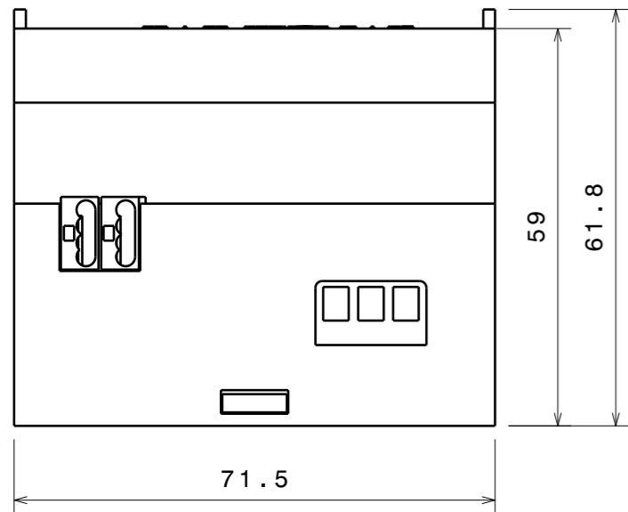
Vista frontale Scala: 1:1
